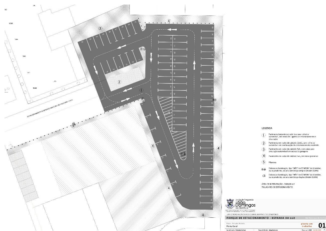
Plano geral intervenção do estacionamento Estrada da Luz
