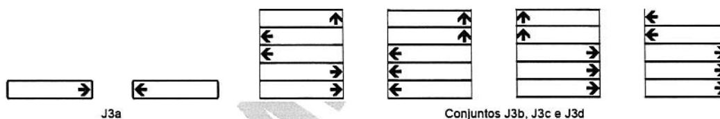
Figura 3. 9 - Colocação vertical de sinais de indicação de âmbito urbano
